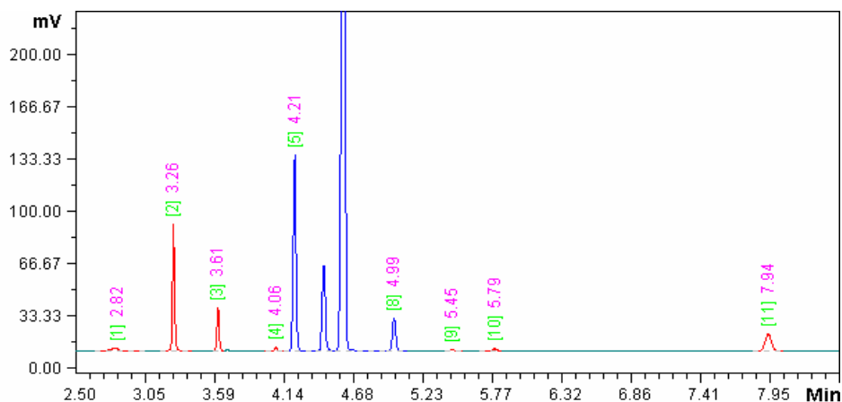
峰 2—二氯甲烷, 峰 3—1, 1-二氯乙烷, 峰 4—三氯甲烷, 峰 5—溴丙烷, 峰 6—1, 2-二氯乙烷, 峰 7—1, 1, 1-三氯乙烷, 峰 8
